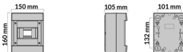
CENTRALINO 4 MODULI SENZA PORTELLO 4 MODULE SWITCHBOARD WITHOUT DOOR
